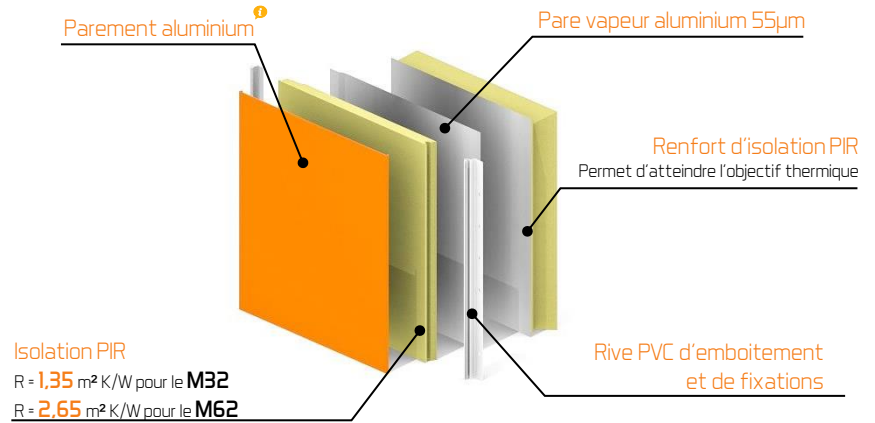
| Vue éclatée du produit Myral |
