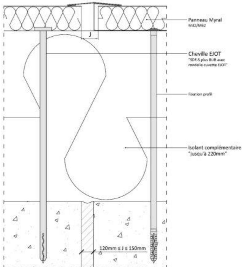
Figure A3 – Détail joint de dilatation de 12 à 15 cm
