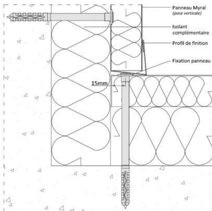
Figure 13b - Angle rentrant – Pose en vêture, lame verticale (coupe horizontale)
