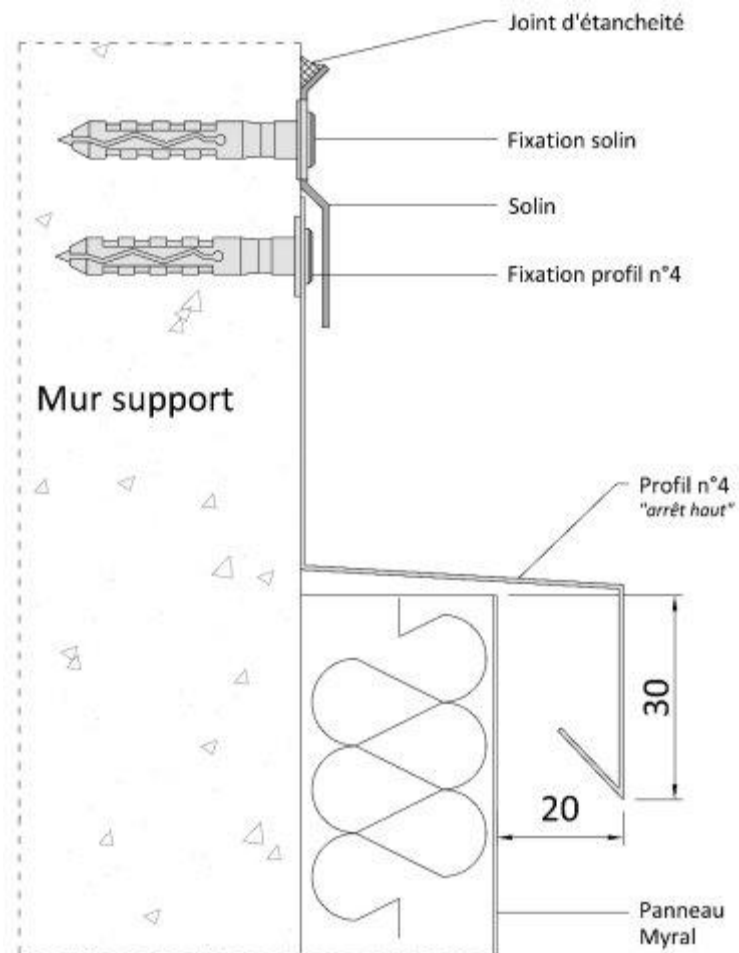
Figure 10a – Haut de façade – Pose en vêtture (coupe verticale)
