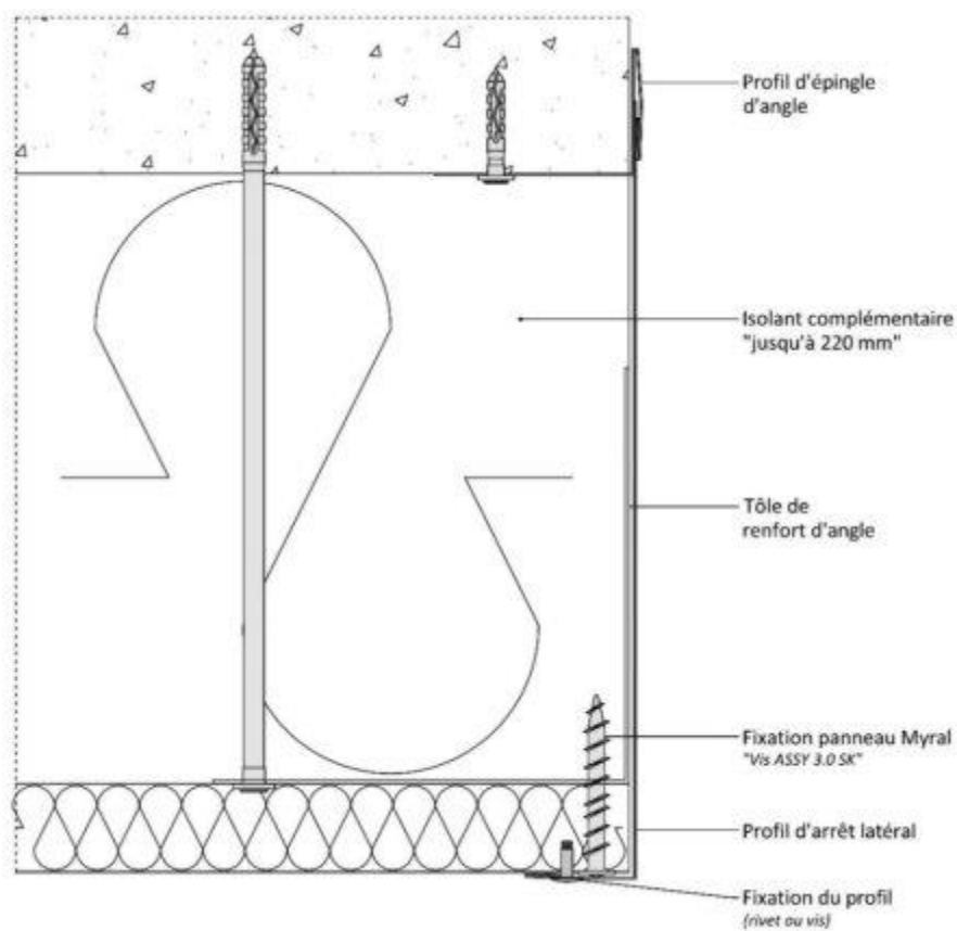
Figure A3 – Détail joint de dilatation de 12 à 15 cm
