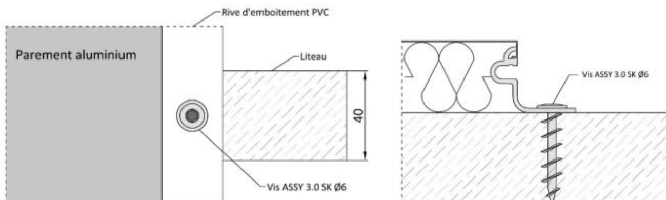
Figure 7b2 – Pose sur tasseaux - Disposition de la vis ASSY 3.0 SK Ø6
