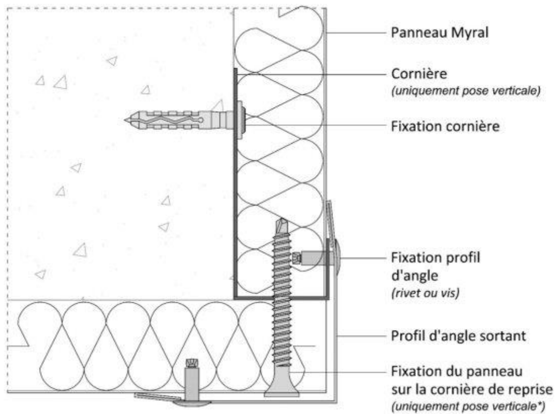
Figure 12b – Angle sortant – Pose en vêtture, lame verticale (coupe horizontale)
