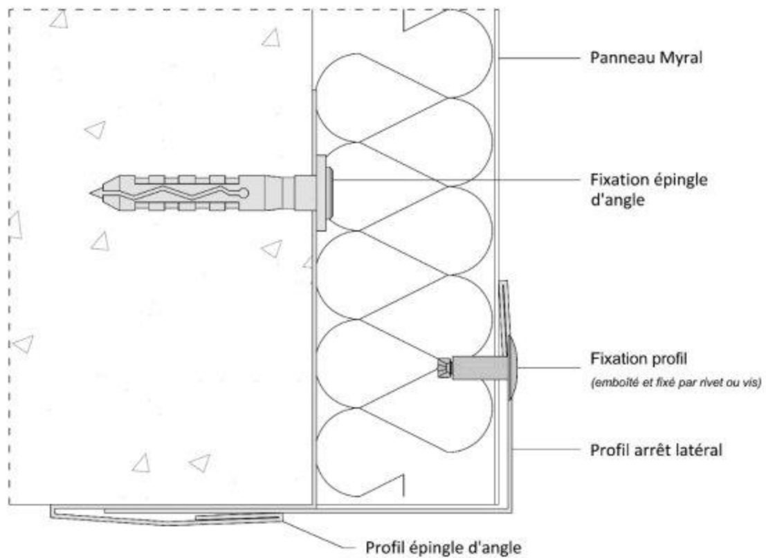
Figure 11 – Angle sortant - Arrêt latéral (coupe horizontale)
