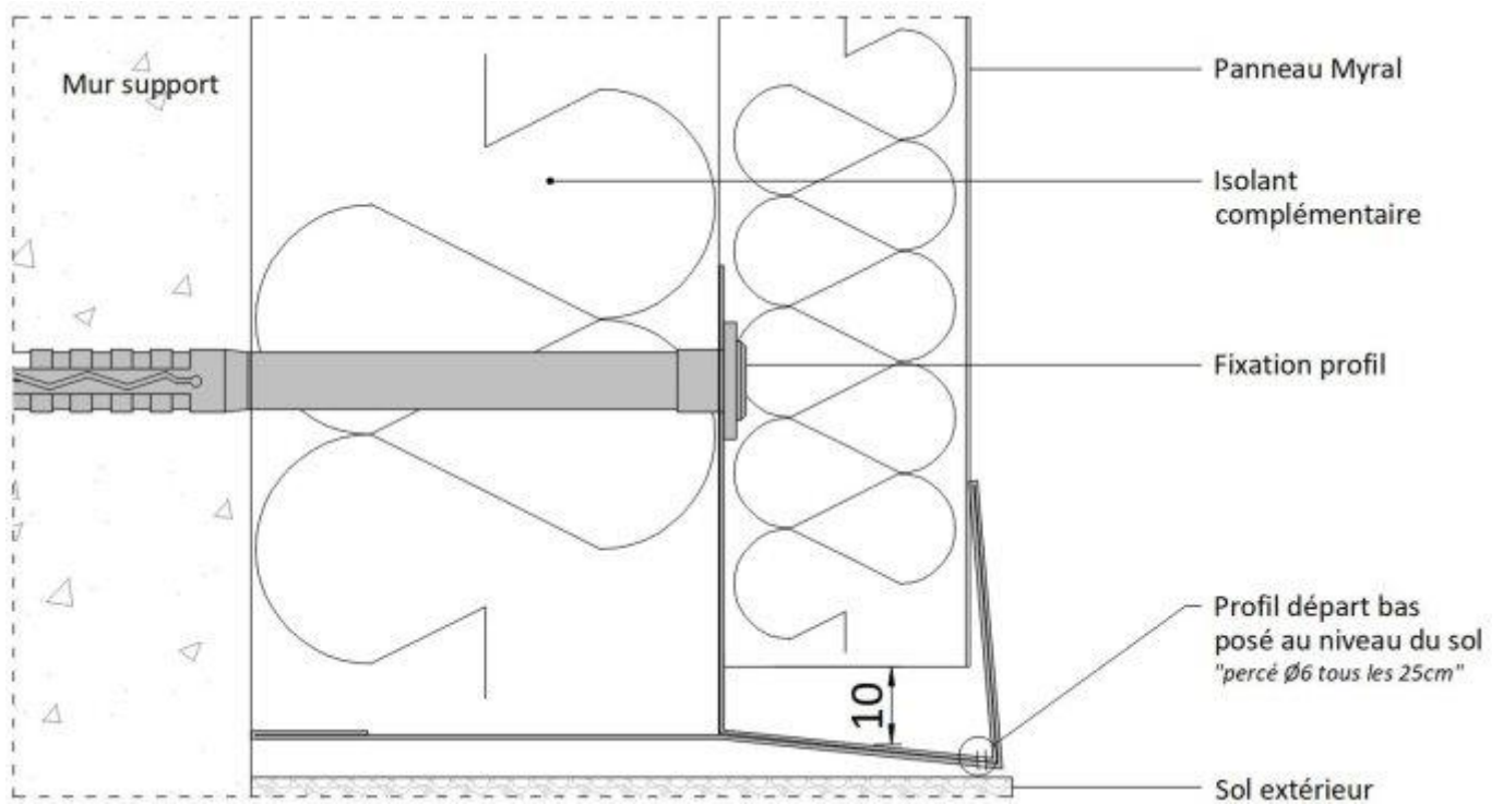
Figure 9b – Bas de façade – Pose en vêture (coupe verticale)
