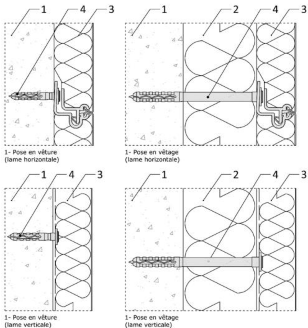
Figure 7a – Fixation des panneaux selon les différentes configurations
