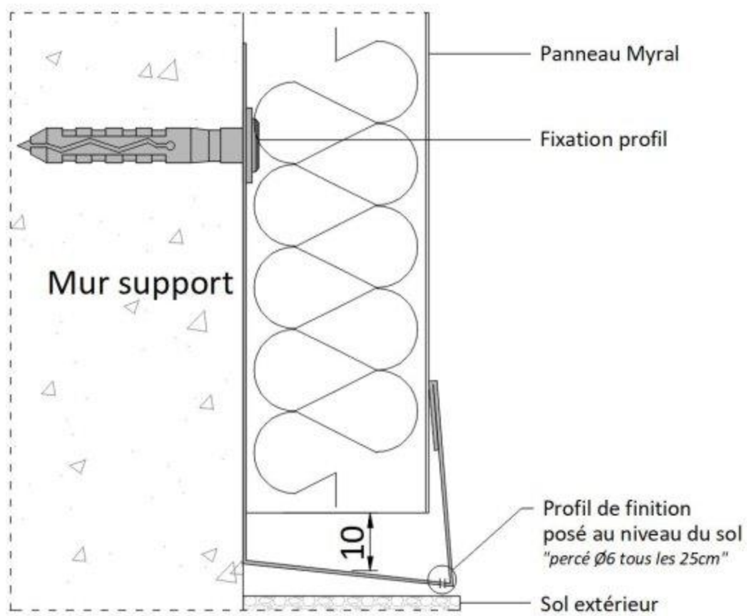
Figure 9a – Bas de façade – Pose en vêture (coupe verticale)
