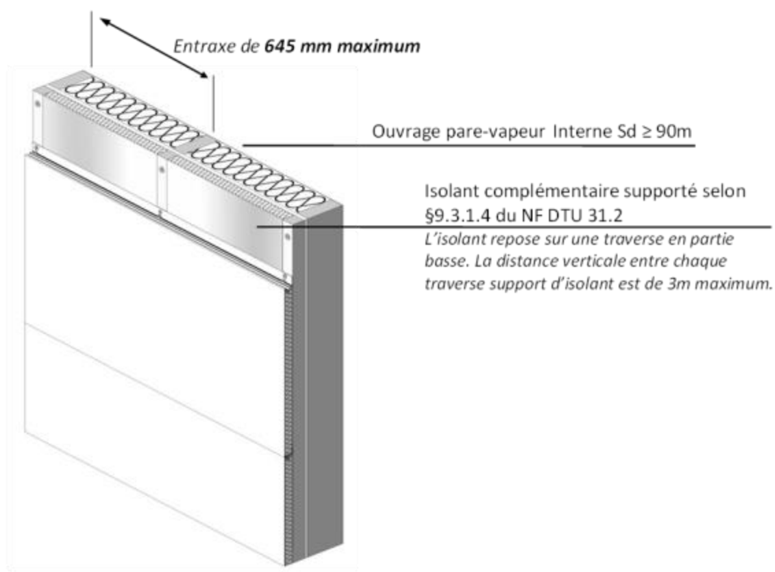
Figure 6b1 – Pose sur tasseaux avec isolant préalable (lames horizontales) sur support COB
