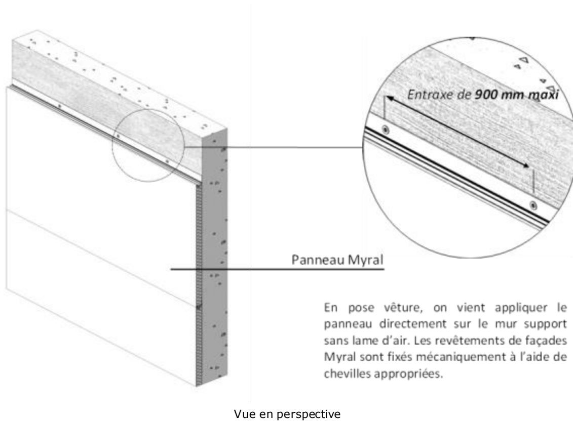
Figure 5a1 – Pose en vêtue (lames horizontales) sur mur béton ou maçonné
