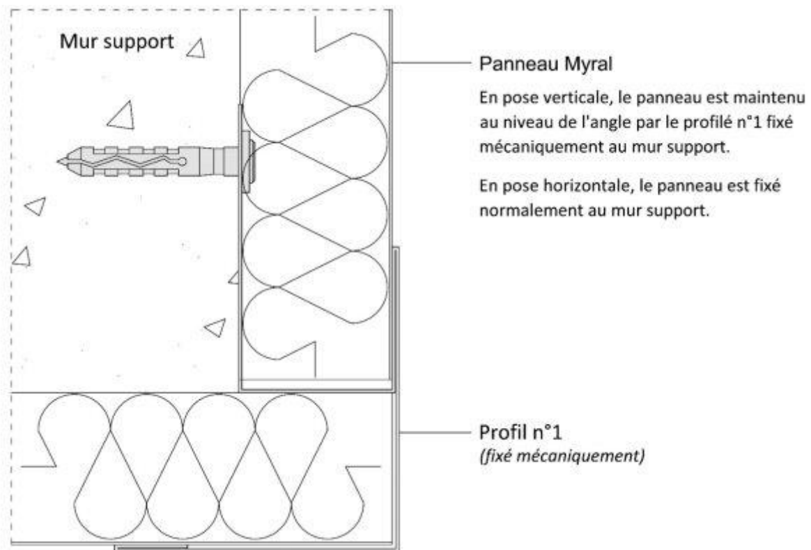
Figure 12a – Angle sortant – Pose en vêtture avec profil n°1, lame verticale (coupe horizontale)
