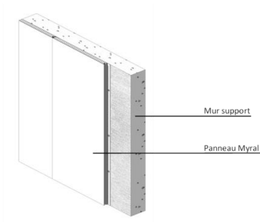
Figure 5a1 – Pose en vêtue (lames horizontales) sur mur béton ou maçonné
