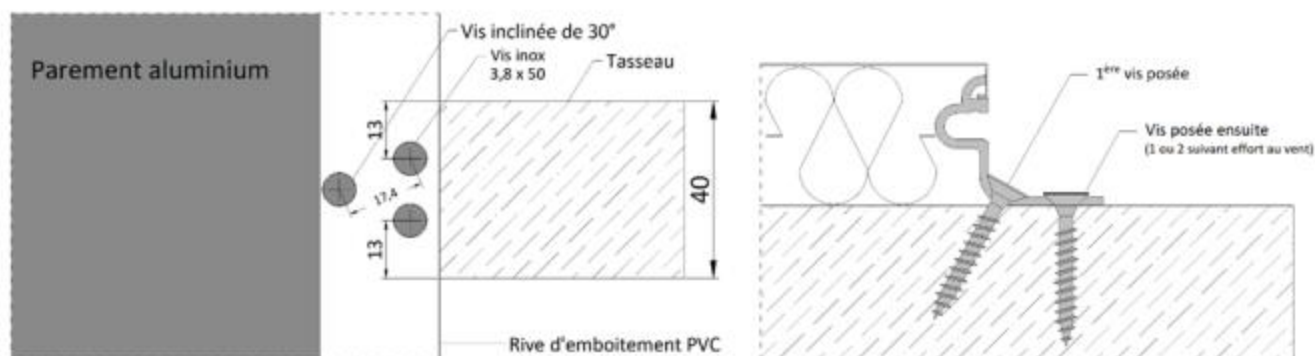
Figure 7b1 – Pose sur tasseaux - Disposition des fixations Ø3,8*25
