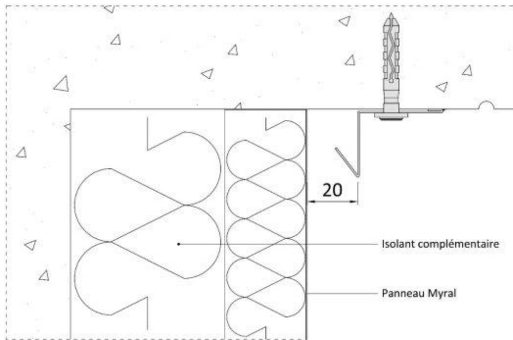
Figure 10c – Haut de façade avec nez de dalle saillant – Pose en vêtage (coupe verticale)
