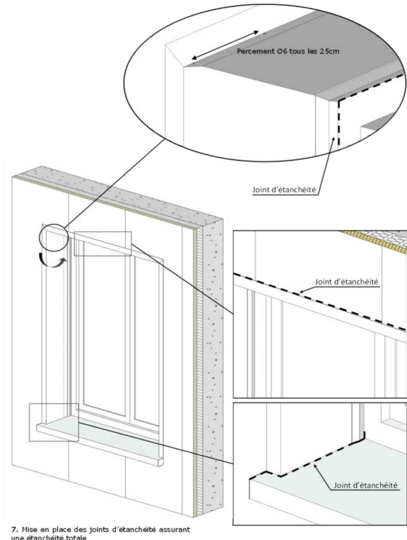
Figure 18- Description de la mise en place des profilés d'ouvertures Vue en perspective
