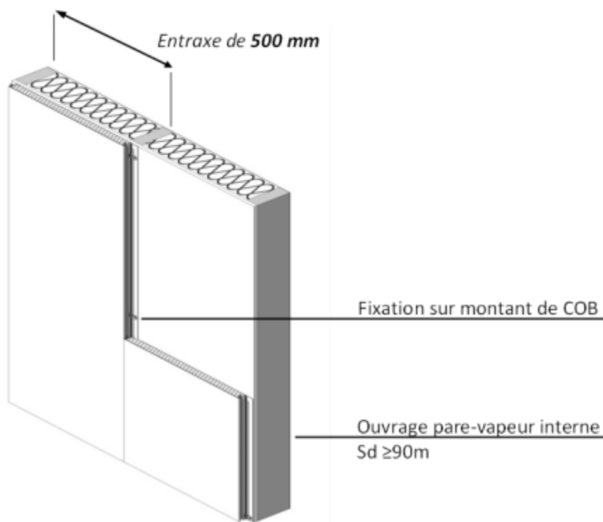
Figure 6a2 – Pose en vêtue (lames verticales) sur support COB
