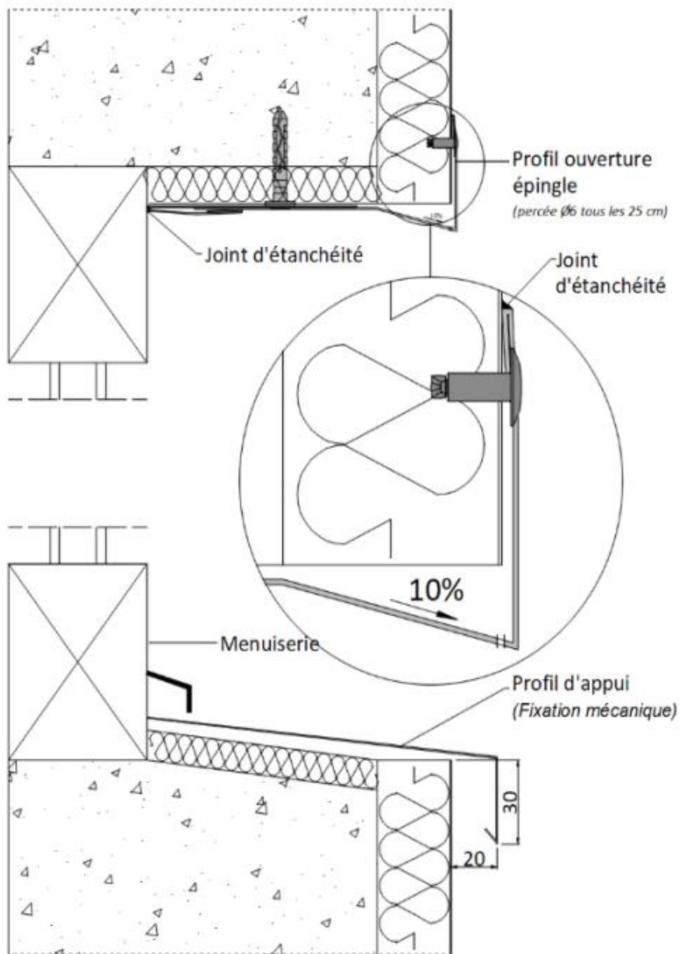
Figure 19b – Habillage de fenêtre – Linteau et appui (coupe verticale)
