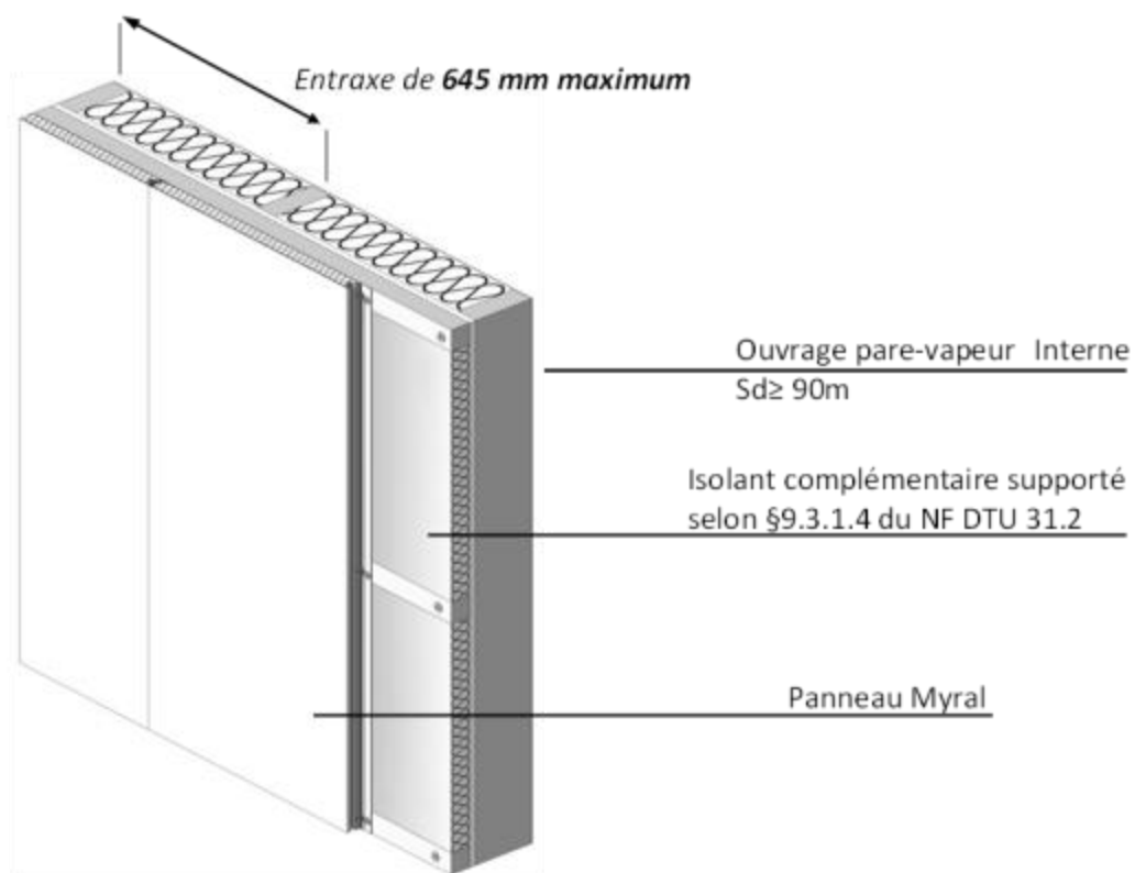
Figure 6b1 – Pose sur tasseaux avec isolant préalable (lames horizontales) sur support COB
