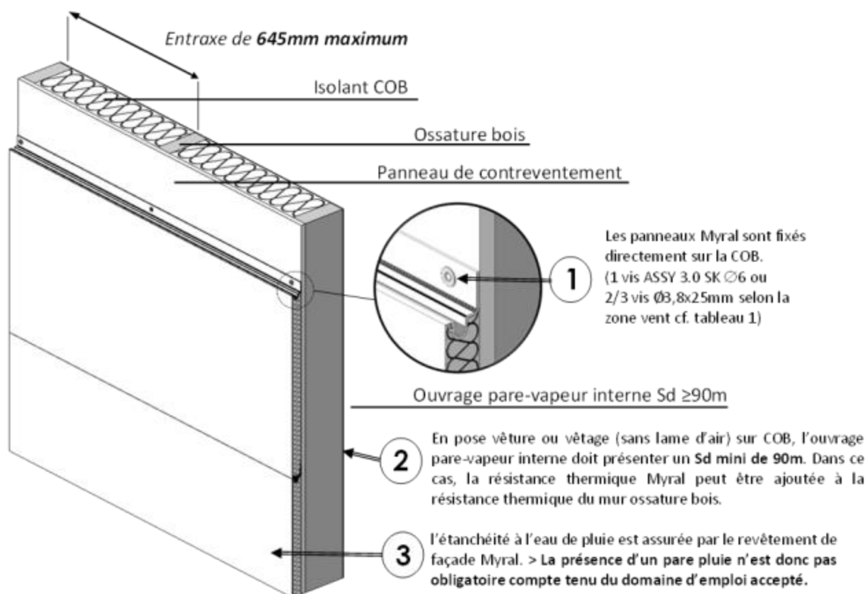
Figure 6a1 – Pose en vêtue (lames horizontales) sur support COB
